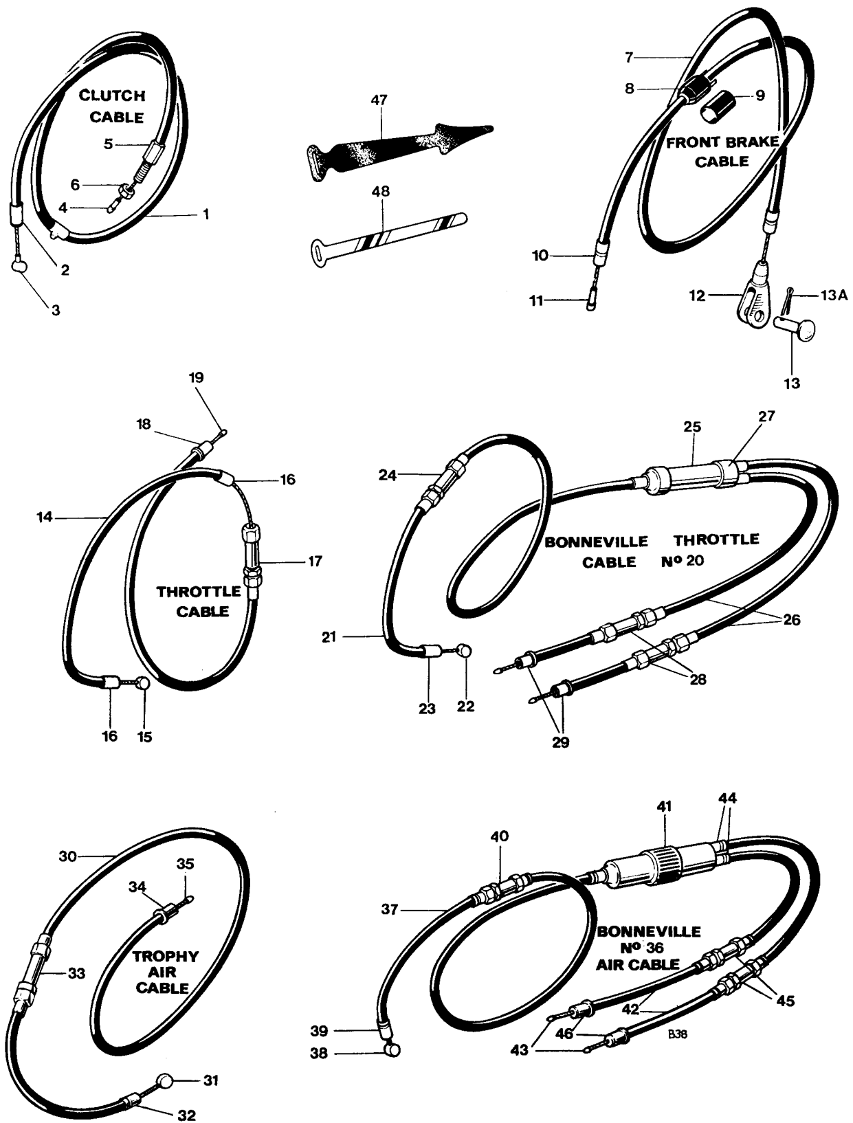
Fig. 27. CONTROL CABLES
